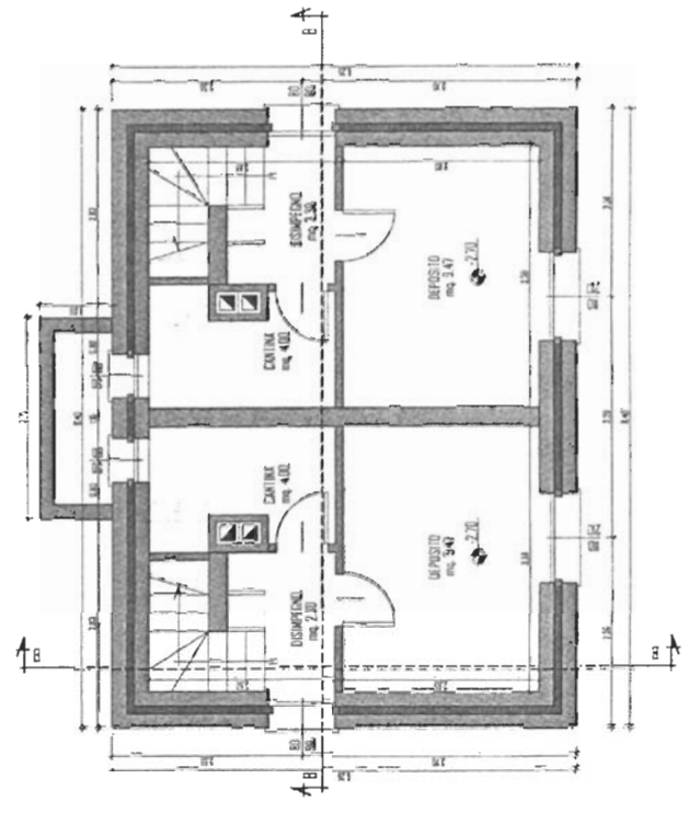
PIANTA PIANO SEMINTERRATO
